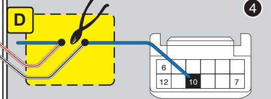
TPMS Module
