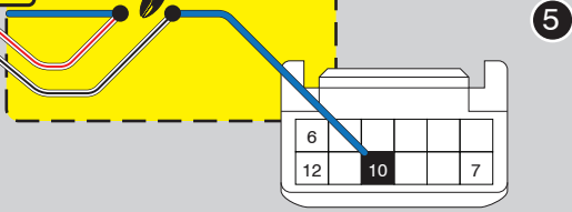
TPMS Module 5
