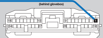
Telematics Module
