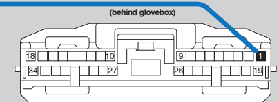
Telematics Module
